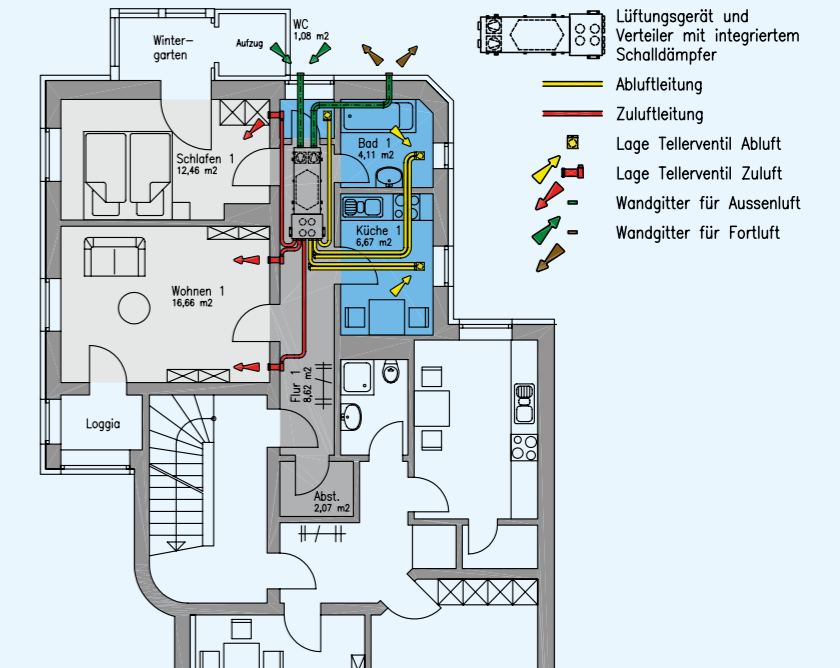
Luftdurchlass innerhalb der später abgehängten Decke
